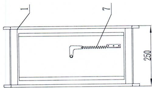
B向视图
