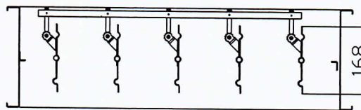
A-A剖视 叶片打开状态
