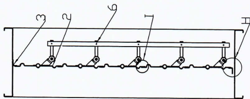
A-A剖视 叶片关闭状态
